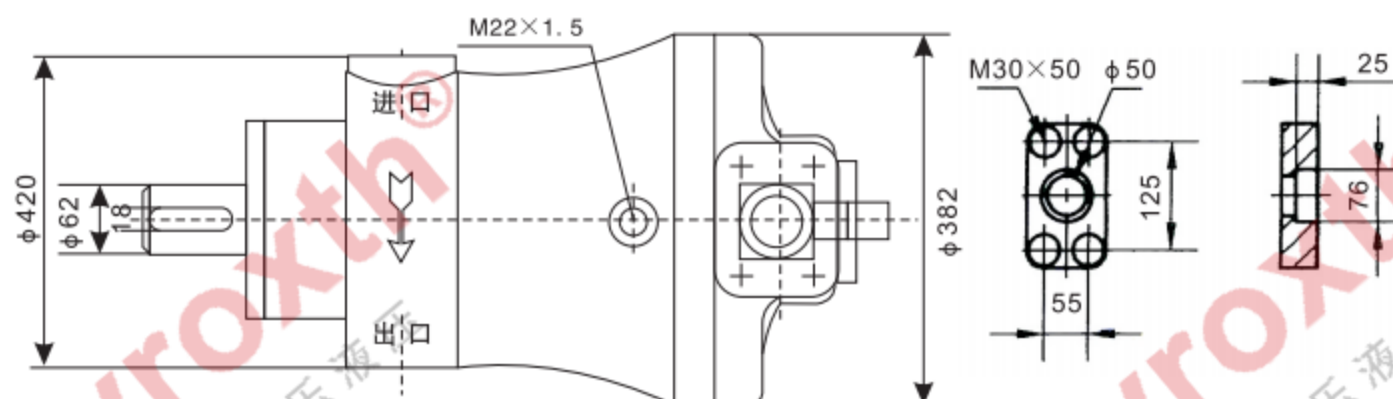
进出口法兰
